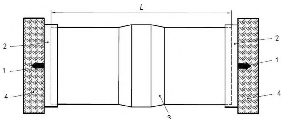
Рисунок 1 – Схема нагружения образцов при продольных нагрузках
