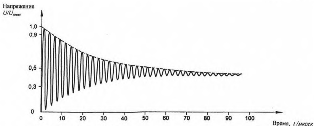
а) T_1/T_2 = 0,8/50 мкс, 370 кГц
