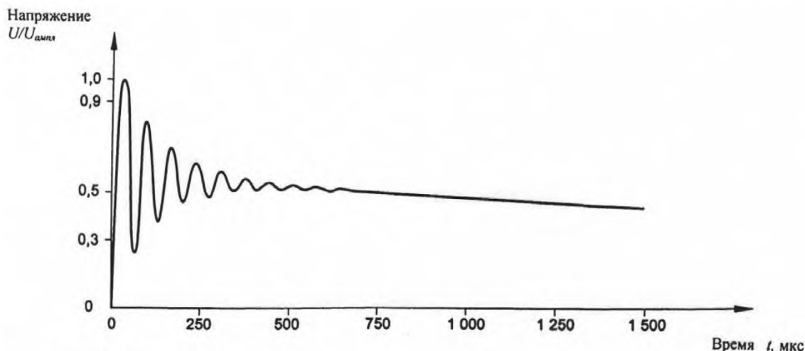
а) T_p / T_2 = 20 / 1\,000 мкс, 15 кГц
