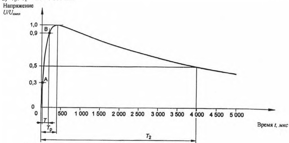
Рисунок 3 - Аперiodический коммутационный импульс
