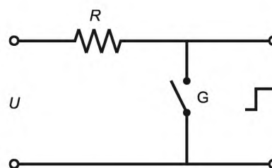
Рисунок В.3,д — Типовая схема цепи ступенчатого генератора
