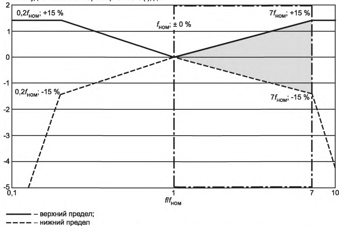
Рисунок 6 — Приемлемая нормализованная амплитудно-частотная характеристика измерительной системы (затемненная область), предназначенной для измерения одной из основных частот f_{\text{НОМ}} (испытанная в диапазоне 1—7 f_{\text{НОМ}} )
