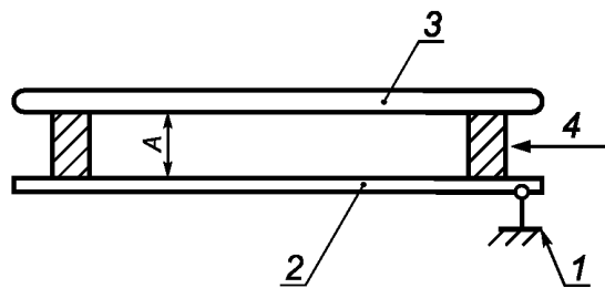
1 — заземление; 2 — заземленная поверхность; 3 — проводящая пластина 150 \times 150 мм; 4 — изолятор
