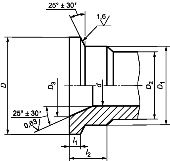
Рисунок 6 — Ниппель неварной
