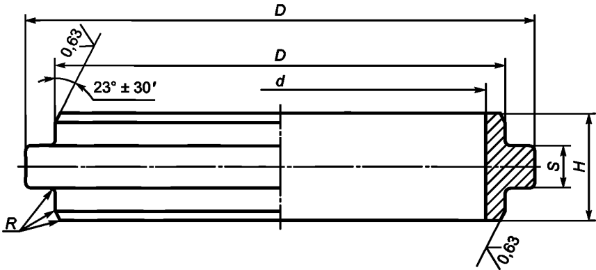
Рисунок 3 — Уплотнительное кольцо
