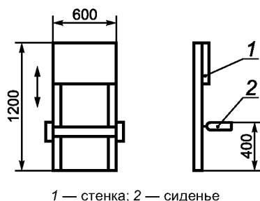
Рисунок Б.1 — Откидное сиденье
