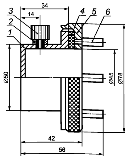
1 — корпус; 2, 4 — прокладка; 3 — винт; 5 — подставка-столик; 6 — стойка
