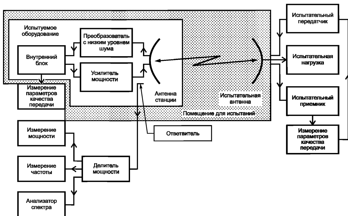
Рисунок 1 — Конфигурация оборудования при испытаниях
