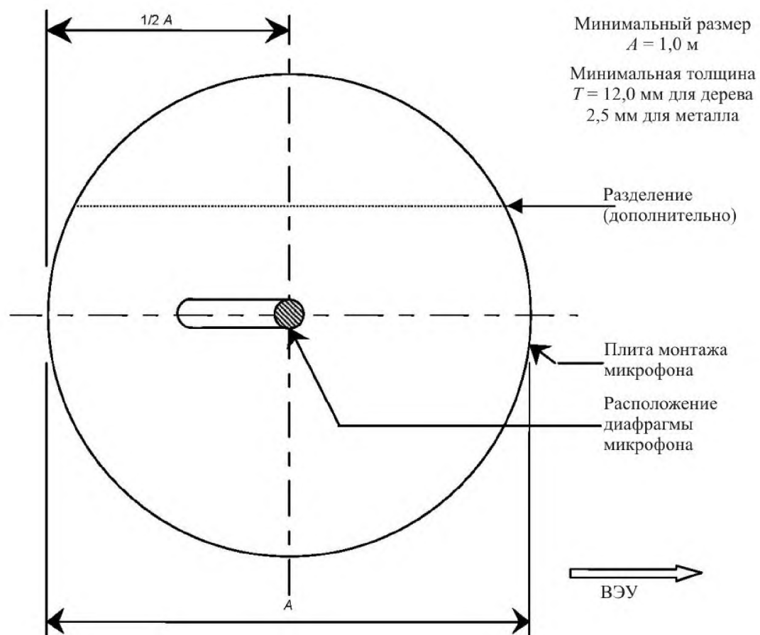
Рисунок 1а – Монтаж микрофона (вид сверху)
