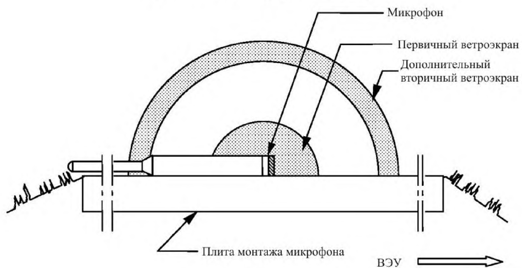
Рисунок 1б – Монтаж микрофона (вид сбоку)
