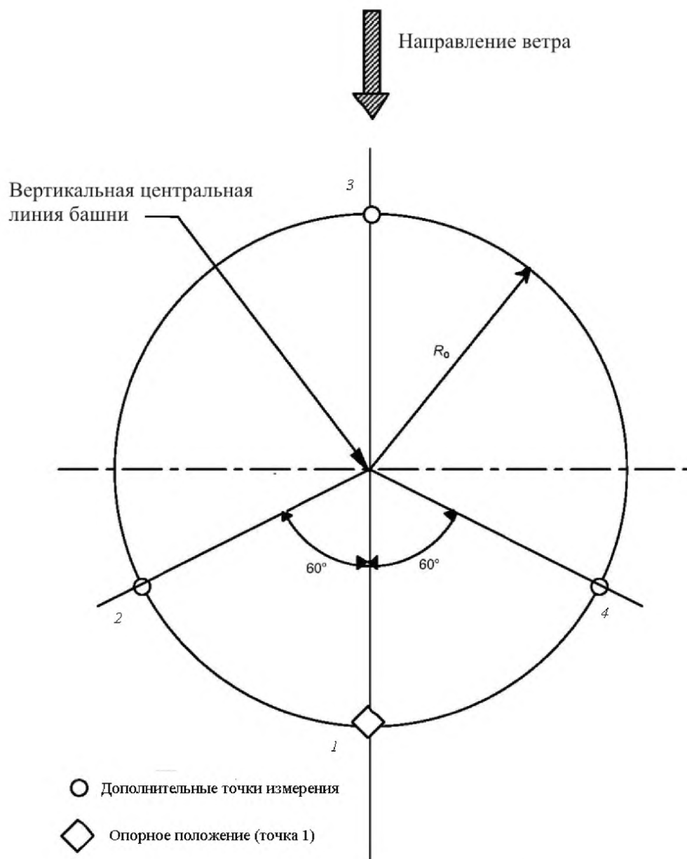
Рисунок 3 – Стандартная схема мест расположения микрофонов (вид сверху)
