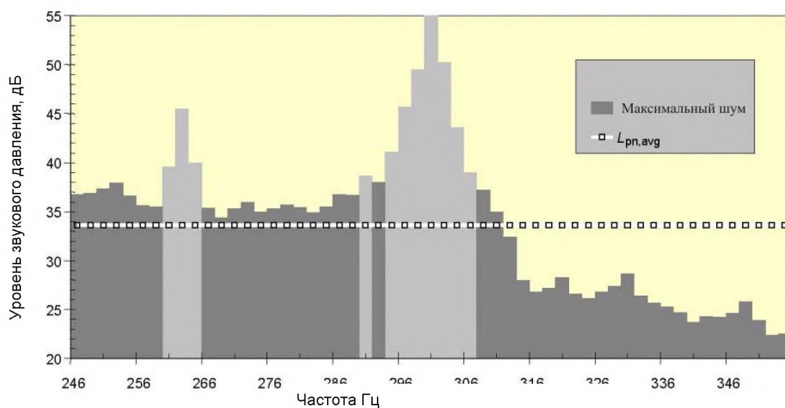
Рисунок 10 – Иллюстрация уровня L_{pn,avg} и линий, классифицируемых как маскирующие
