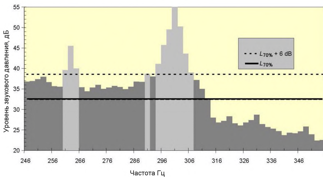
Рисунок 9 – Иллюстрация линий ниже критерия L_{70\%} + 6 \text{ dB}
