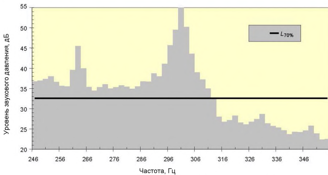
Рисунок 8 – Иллюстрация уровня L_{70\%} в критичной полосе частот
