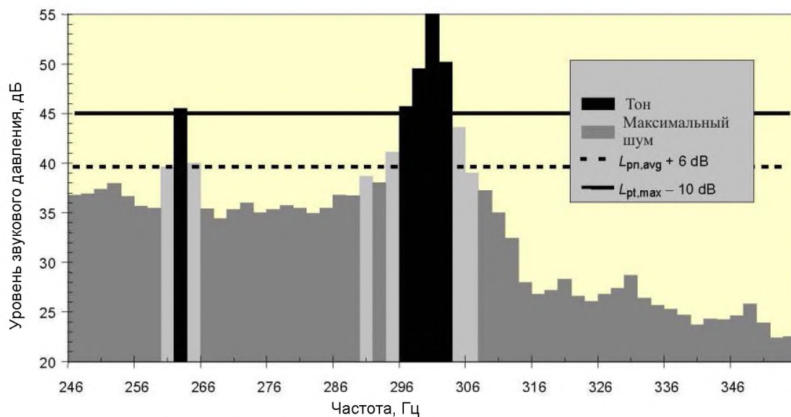
Рисунок 11 – Иллюстрация классификации всех спектральных линий
