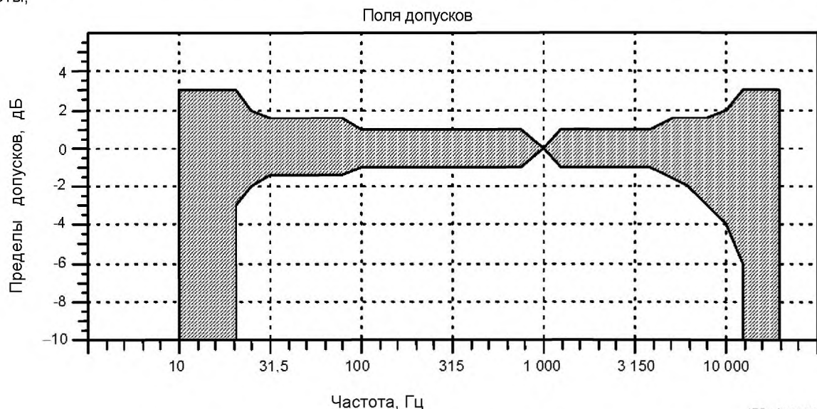
Рисунок В.1 – Допуска для частотной характеристики, по [7], тип 1
