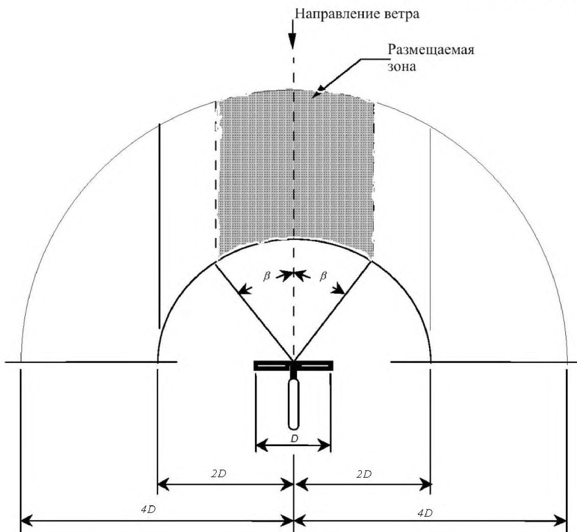
Рисунок 5 – Размещения метеорологической вышки как функция от \beta – вид сверху
