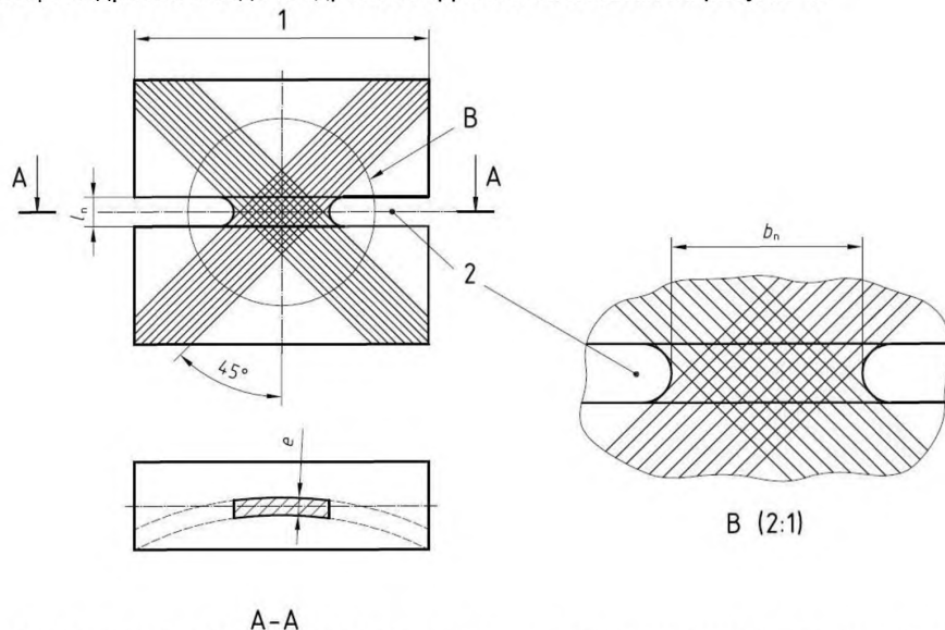
А – А 1 – края образца трубы; 2 – область надреза; l_n – расстояние между зажимами; b_n – ширина образца в месте сужения; e – толщина стенки трубы
