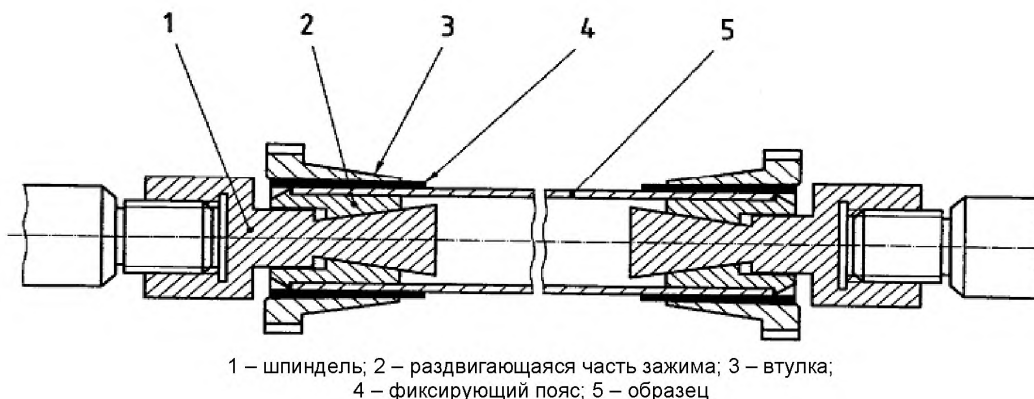
Рисунок 1 – Зажим для крепления образца (для метода Б)
