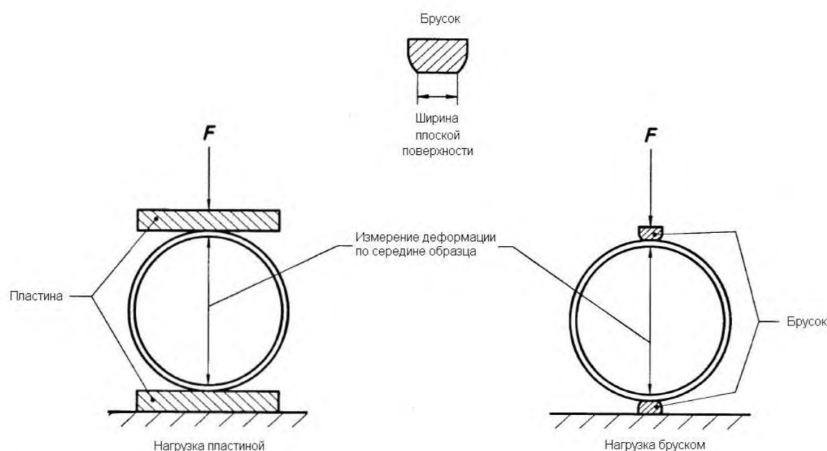
Рисунок 2 – Схема установки испытываемого образца в опорных площадках
