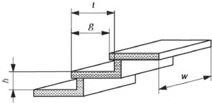
Рисунок 4 – Размерные параметры для лестниц и наклонных лестниц
