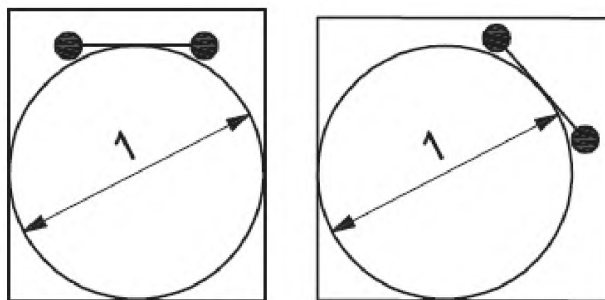
1– внутренний диаметр ограждения
