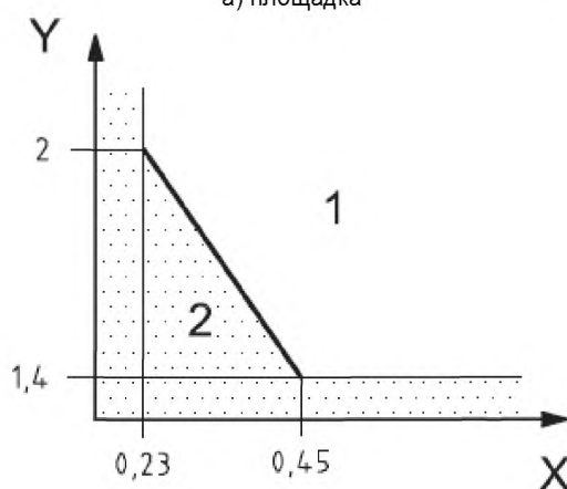
б) проход и наклонный проход
