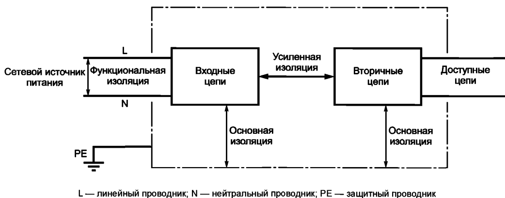
Рисунок 5a — Пример 1 — Упрощенная схема изоляционной системы, содержащей функциональную, основную и усиленную/двойную изоляцию для оборудования класса I
