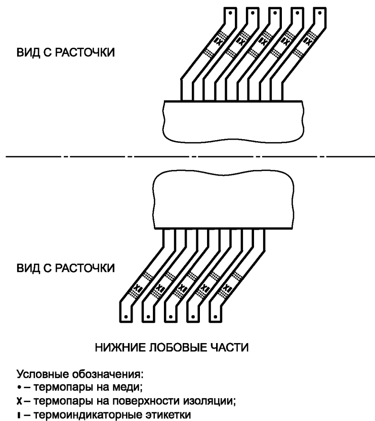
Рисунок Г.2 — Схема установки термопар и ТЭ на лобовых частях обмотки статора гидрогенератора
