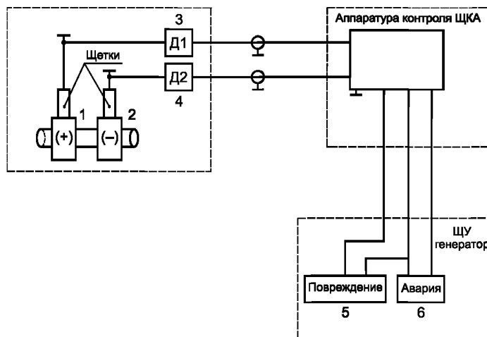
Рисунок М.2 — Схема подключения аппаратуры к ЦКА и панели управления гидрогенератором
