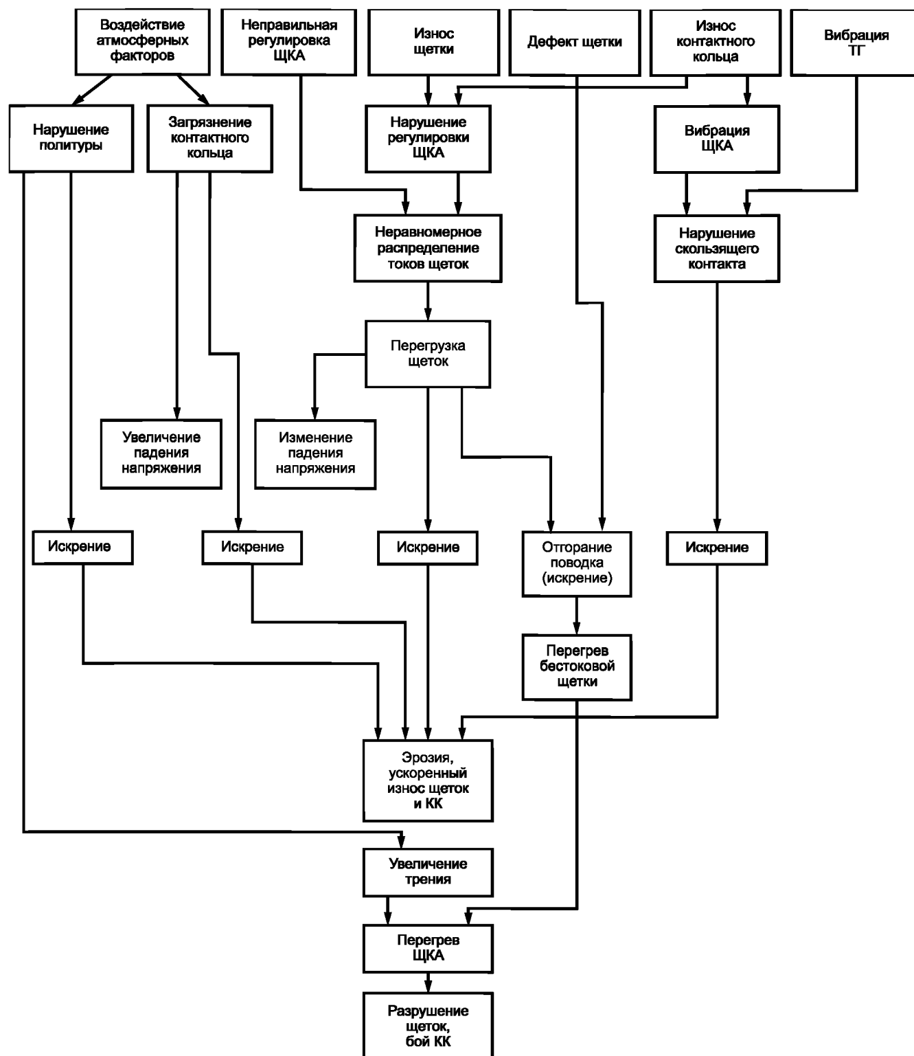
Рисунок М.1 — Сценарии развития дефектов ЩКА
