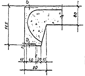
Деталь "Ж"
