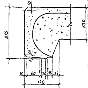
Деталь "Ж"
