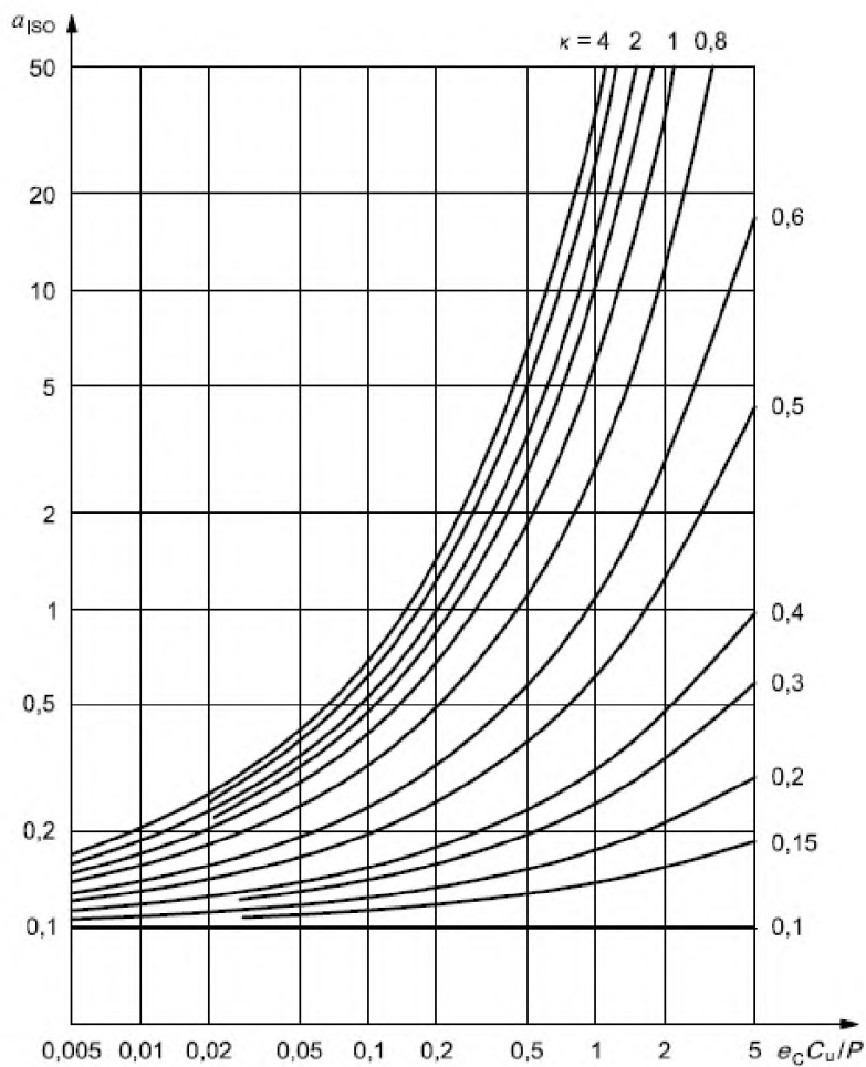
Рисунок 4 — Коэффициент модификации ресурса, a_{\text{ISO}} , для радиальных и радиально-упорных роликовых подшипников
