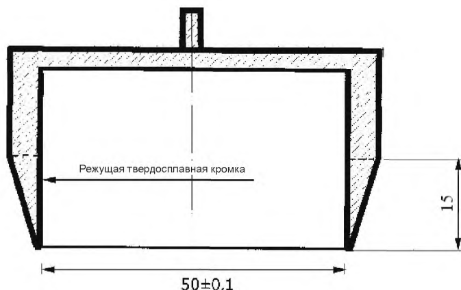
Рисунок 2 — Сверло-коронка с режущей твердосплавной кромкой
