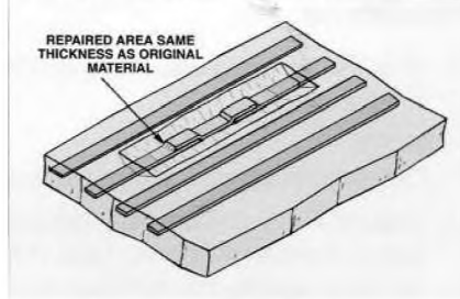
Рисунок 24 h – Герметизация отреставрированного участка
