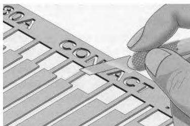
Рисунок 35 с – Вырезание нового концевого контакта
