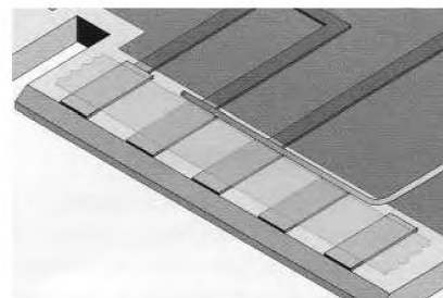
Рисунок 36 d – Припаивание провода по кромке металлизуемых концевых контактов
