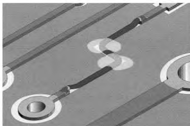
Рисунок 21 е – Приклеивание провода к поверхности платы клеем
