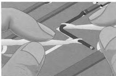
Рисунок 21 с – Придание проводу необходимой формы
