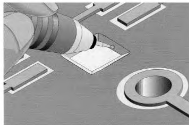
Рисунок 10 b – Выравнивание кромки ручной дрелью или надфилем
