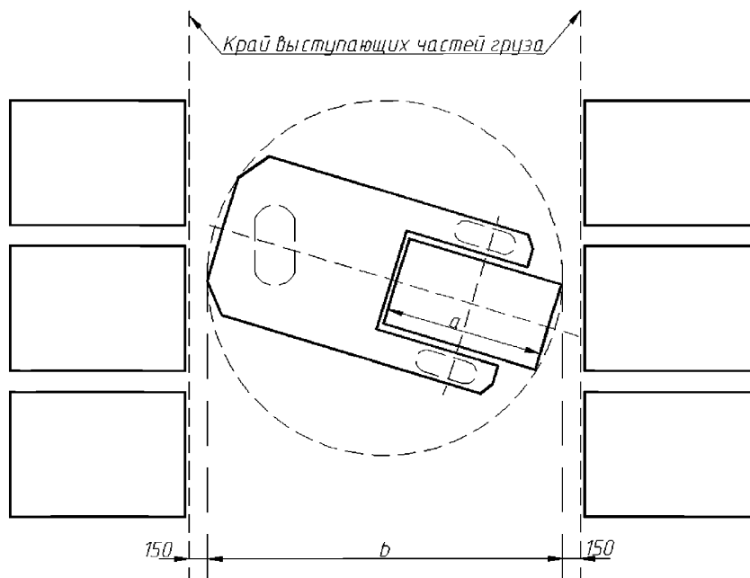
Рисунок 4 – Параметры зазора между ШТ и грузами
