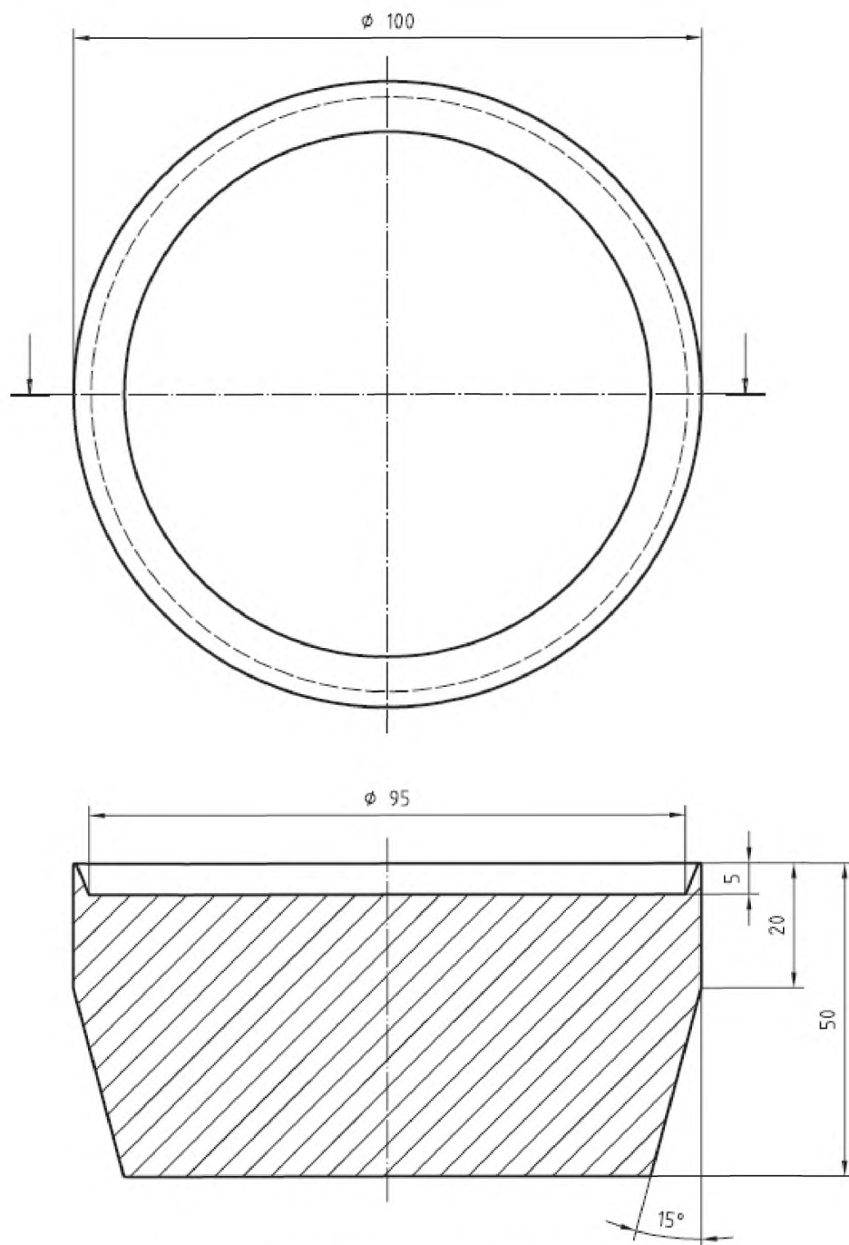
Рисунок 5 – Дополнительное устройство для установки проб
