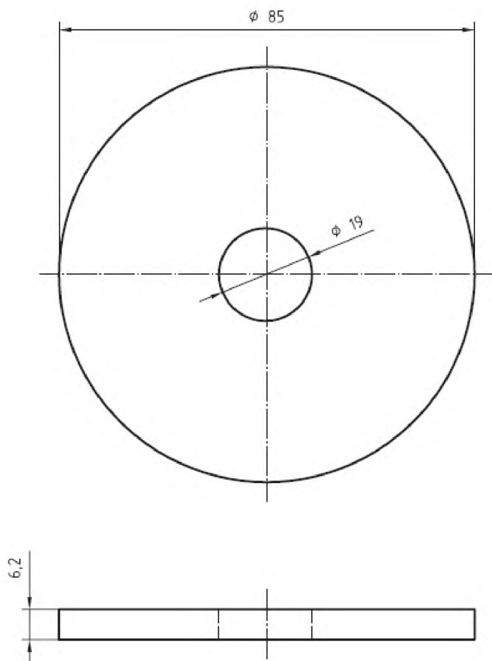
Рисунок 4 – Дополнительный груз
