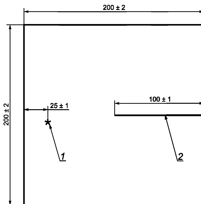
1 — отметка конца длины разрыва; 2 — надрез
