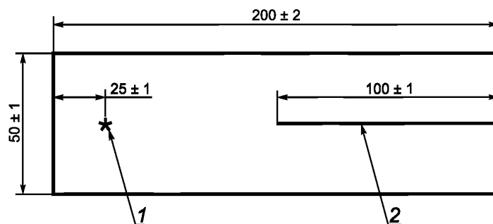
1 — отметка конца разрыва; 2 — надрез
