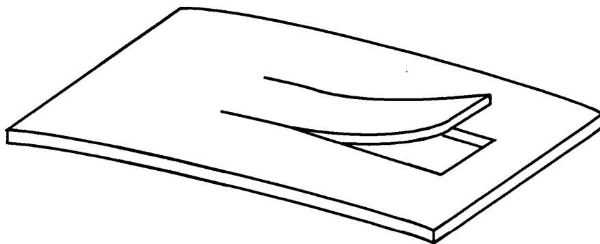
Рисунок 1– Пример испытуемого образца в форме языка
