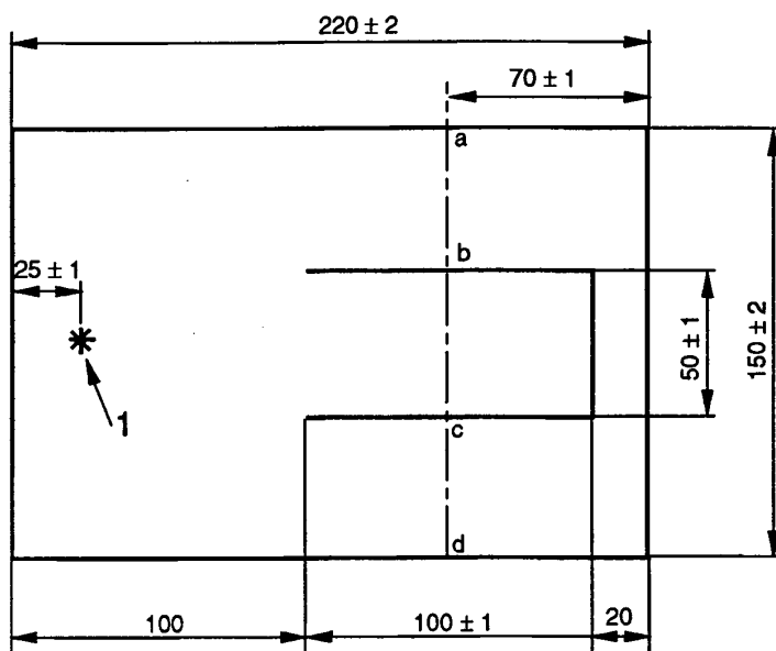
Рисунок 2 – Испытуемый образец в форме языка
