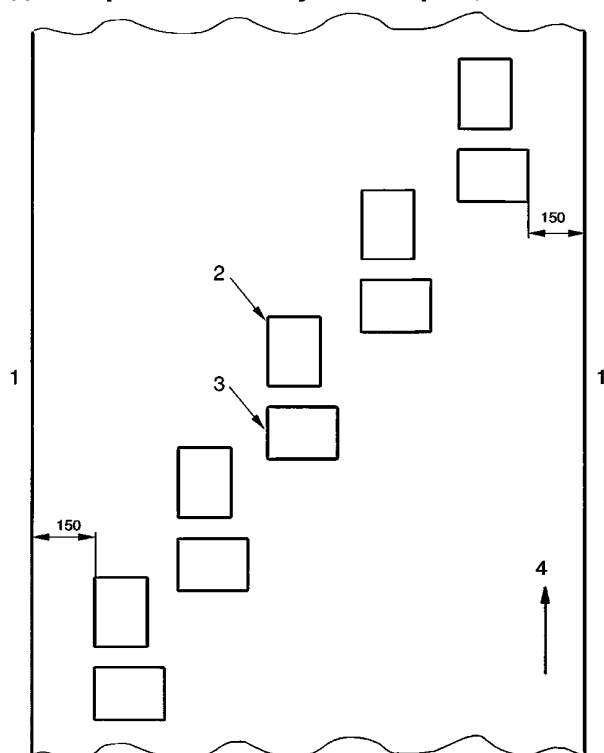
1 – край; 2 – пробы для раздирания «поперек основы»; 3 – пробы для раздирания «поперек утка»; 4 – основа Рисунок В.1
