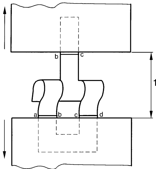
Рисунок 3 — Расположение зажимов
