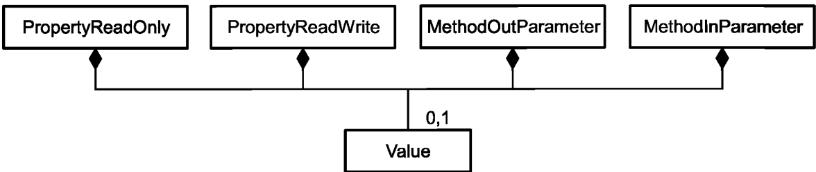
Рисунок C.2 — Элемент Value для несвязанных определений типа
