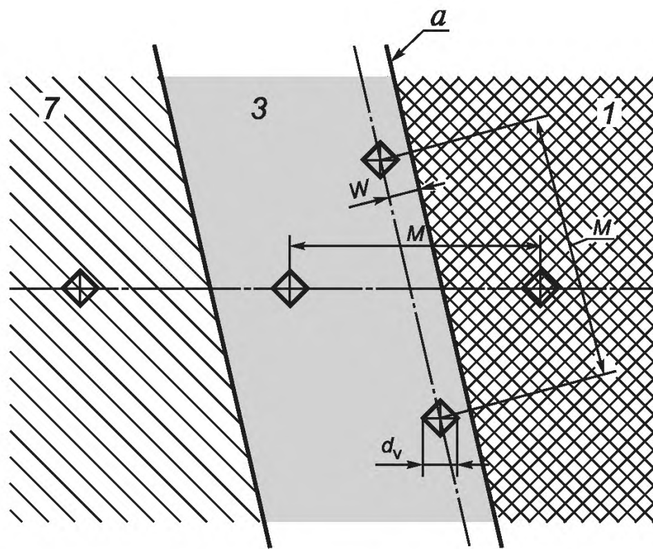
а) Твердость по Виккерсу ( d_V/2 \leq W \leq d_V )
