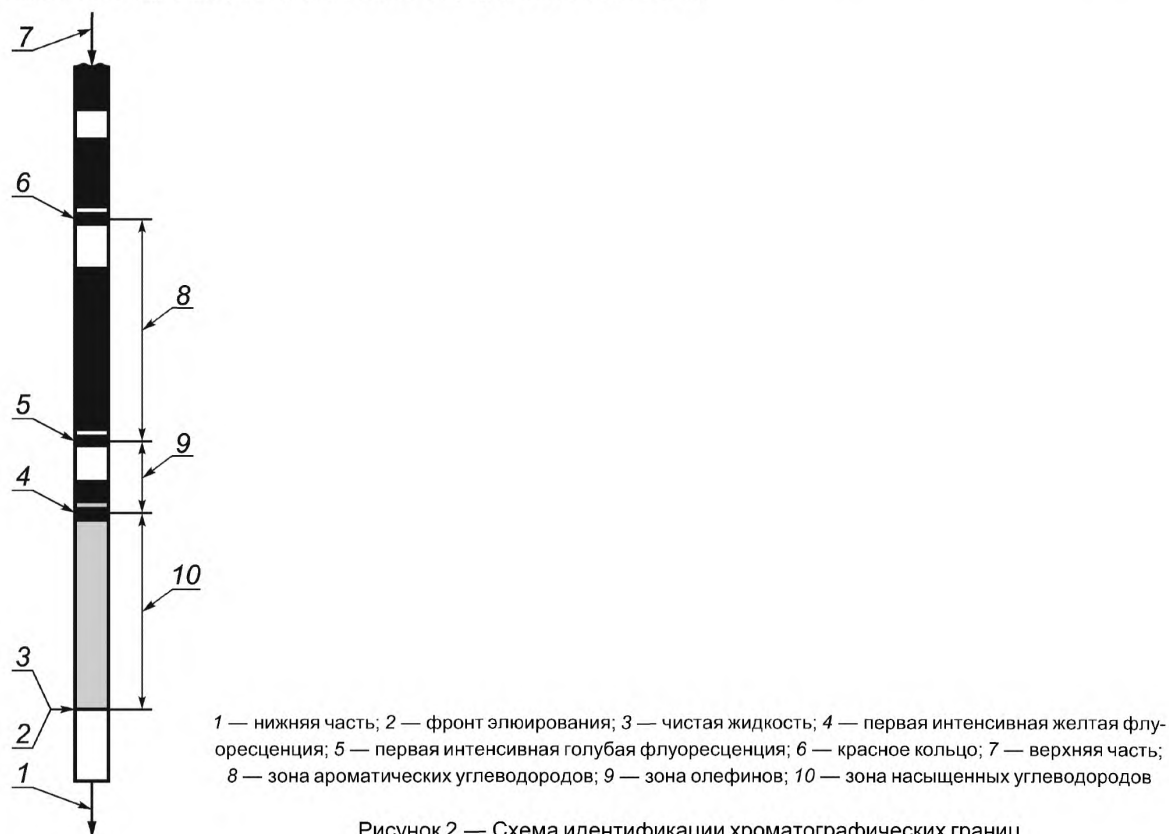
Рисунок 2 — Схема идентификации хроматографических границ
