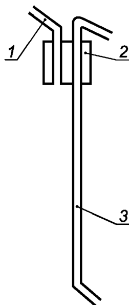
1 — трубка для налива; 2 — пробка; 3 — пробоотборная трубка
