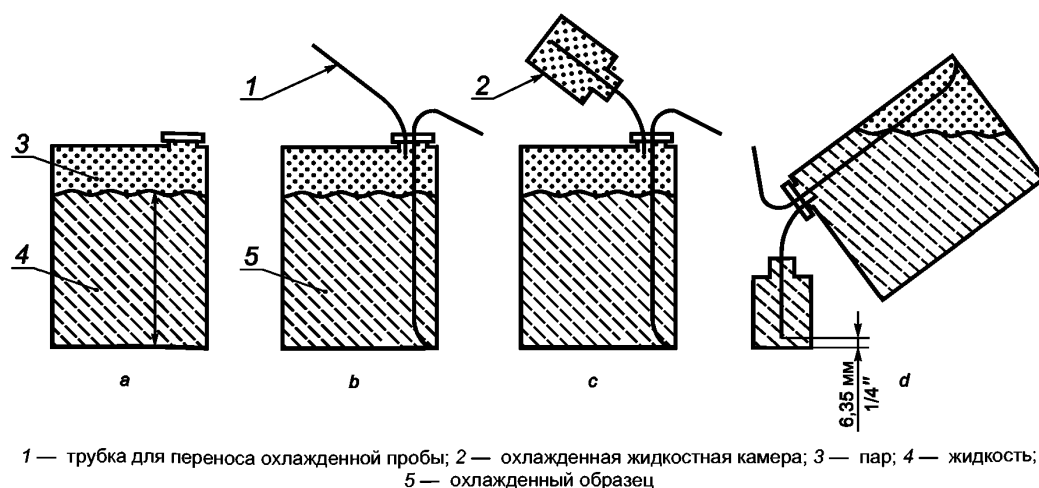
Рисунок 1 — Упрощенная схема способа переноса пробы в жидкостную камеру контейнера открытого типа
