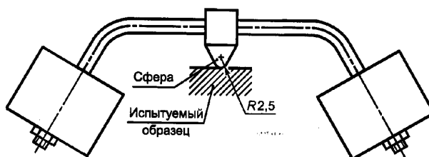
Рисунок 1 – Установка для испытания на теплостойкость
