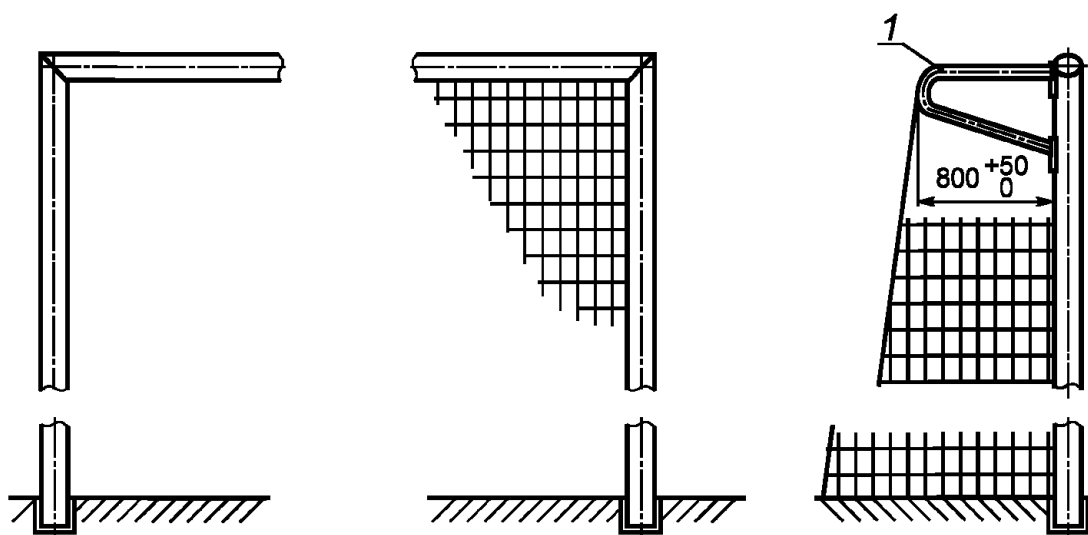
1 — консоль для натяжения сетки
