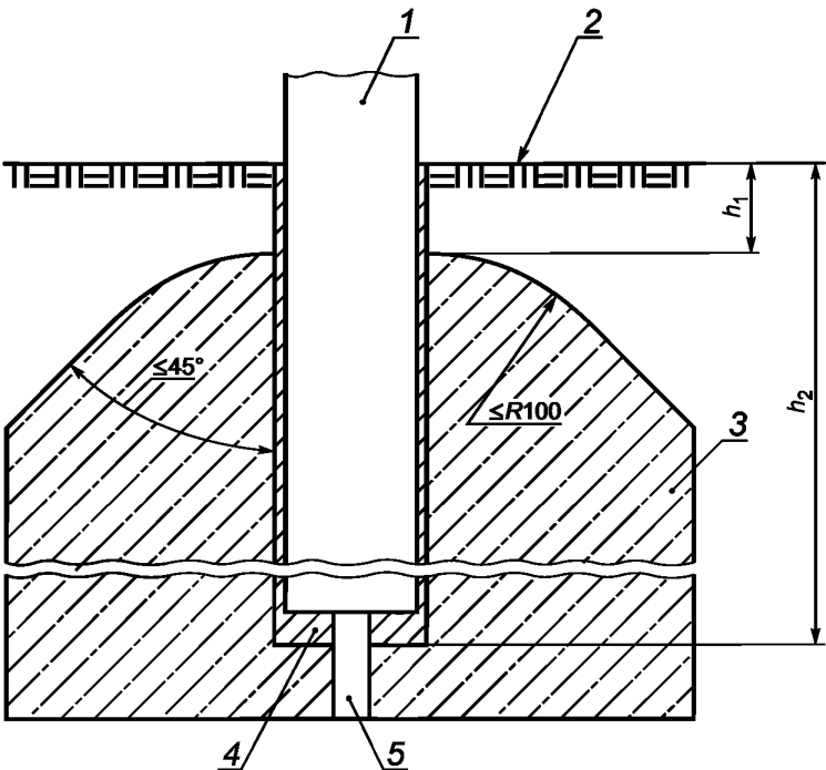
1 — штанга/стойка натяжения сетки; 2 — покрытие футбольного поля; 3 — бетон; 4 — установочная гильза; 5 — дренажное отверстие
