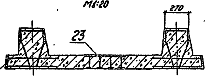
6-6 М1:20
