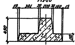
6-6 М1:20
