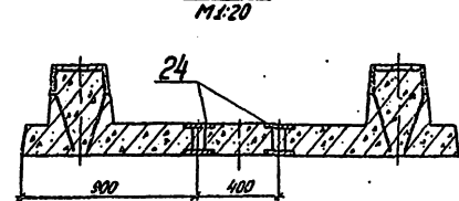
7-7 М1:20
