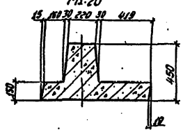
8-8 М1:20
