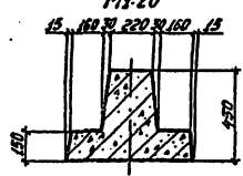
7-7 М1:20
