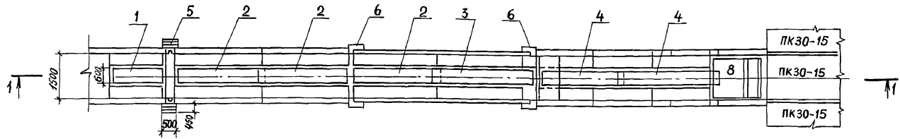
Деталь армирования шероховатости быстротока.
