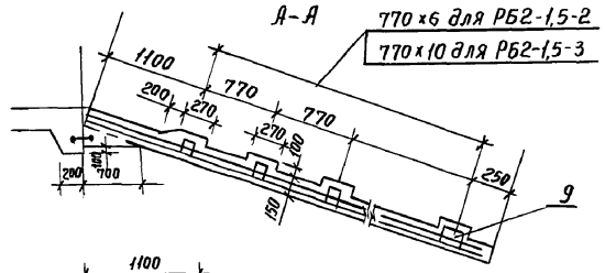
Деталь армирования шероховатости быстротока
