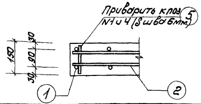
Деталь установки монтажной петли
