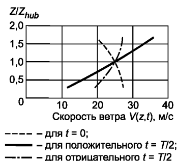
Профиль ветра до начала сдвига ( t = 0 , штриховая линия) и при наибольшем сдвиге ( t = 6 с, сплошная линия)
