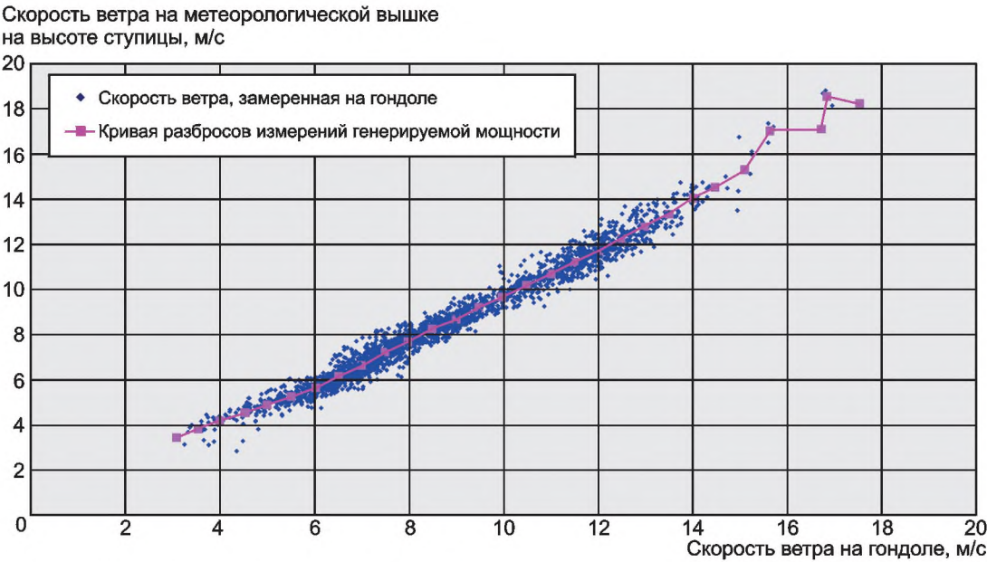
Рисунок 2 — Пример представления данных по передаточной функции, получаемой в соответствии с приложением Г
