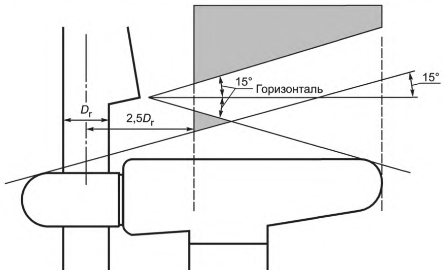
Рисунок А.1 — Установка анемометра на вершине гондолы
