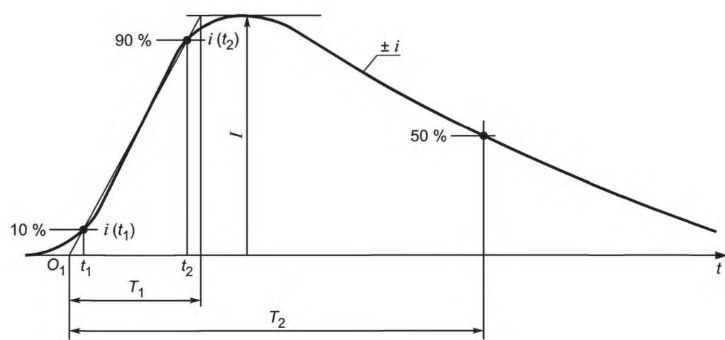
O_1 — виртуальное начало координат; I — пиковый ток; i — ток; t — время; T_1 — время нарастания импульса; T_2 — время до половины значения
