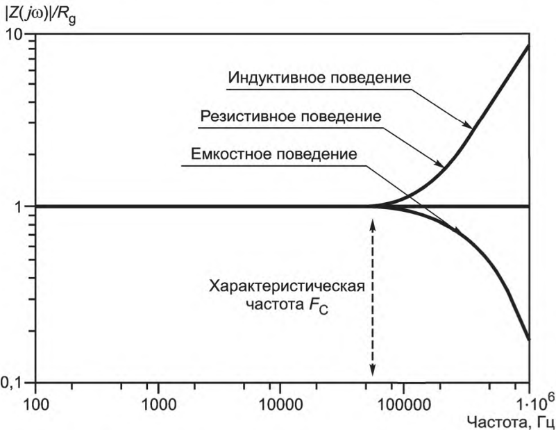
Рисунок 1.2 — Зависимость частоты от полного сопротивления заземления
