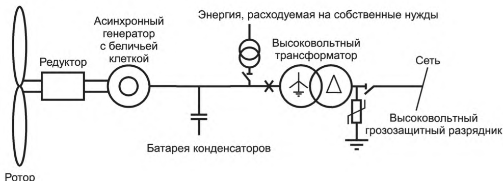
Рисунок 4а — асинхронный генератор с беличьей клеткой
