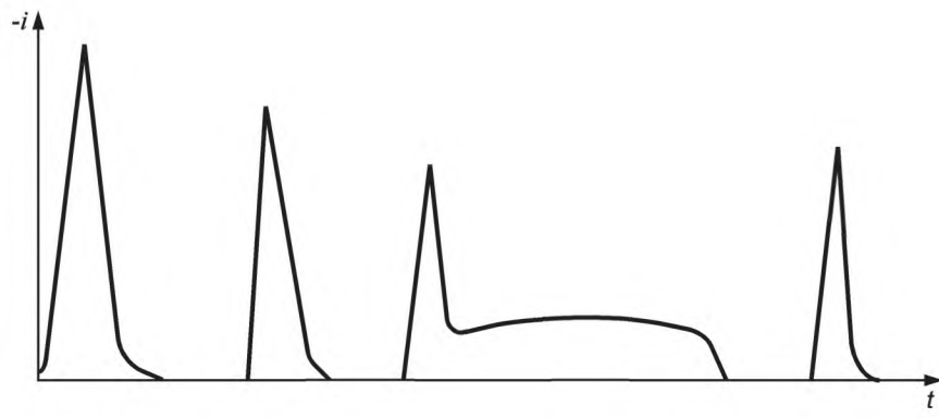
Рисунок А.2 — Характерный профиль отрицательной вспышки «грозовая туча — земля» (не в масштабе)
