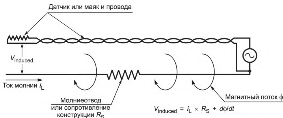
Рисунок С.3 — Индуктированные молнией напряжения между молниеотводом или конструкцией и проводами датчика
