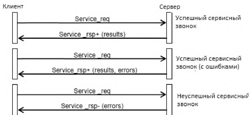
Рисунок 9 - Циклограмма
