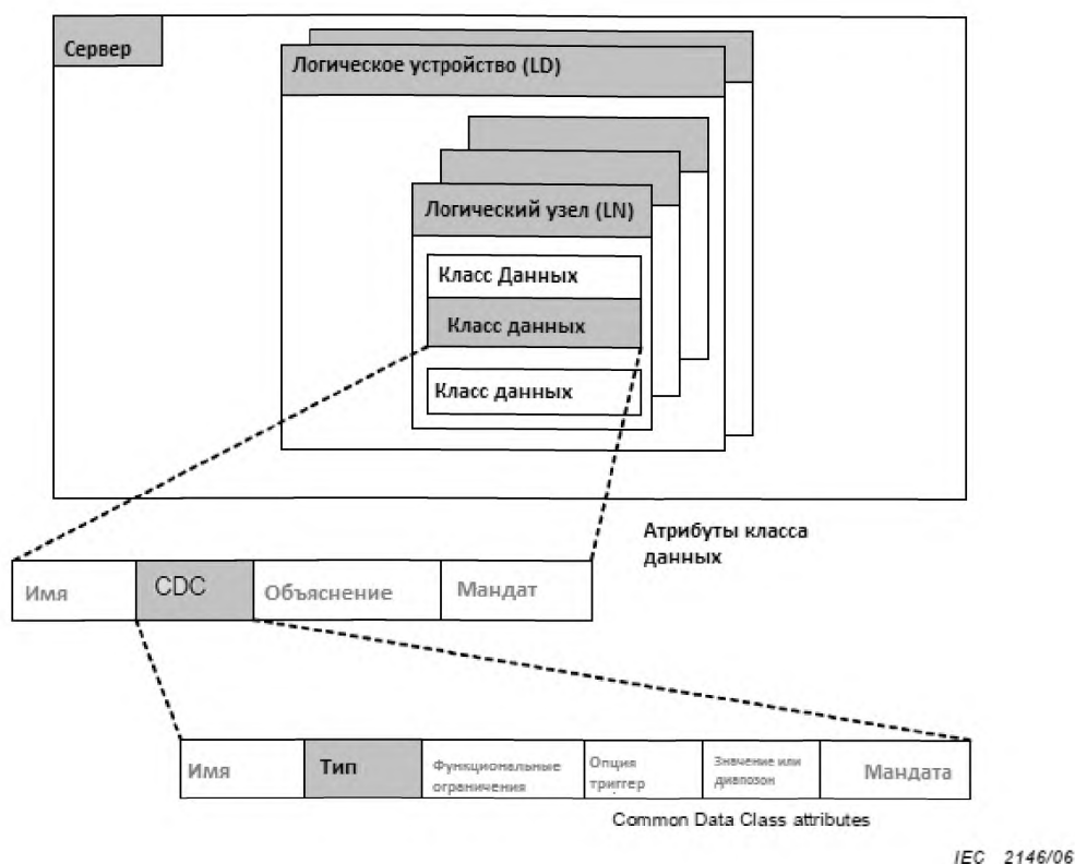
Рисунок 4 – Структура информационной модели ВЭС
