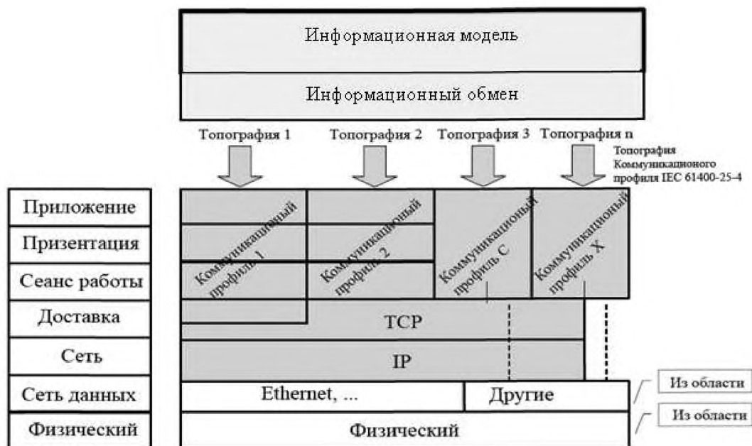
Рисунок 11 – Коммуникационные профили
