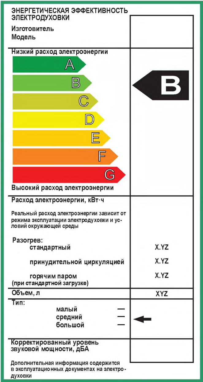
Рисунок А.1 — Маркировка эффективности электрошкафа
