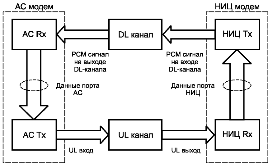
Рисунок В.1 — Общая схема функционирования тональных модемов
