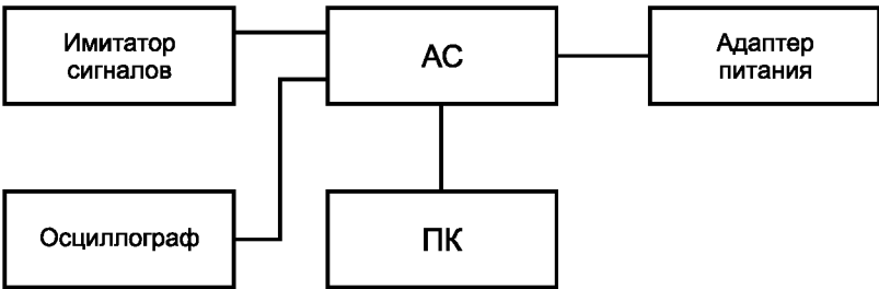
Рисунок Д.4 — Схема испытательного стенда
