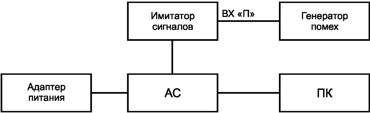
Рисунок Д.5 — Схема испытательного стенда
