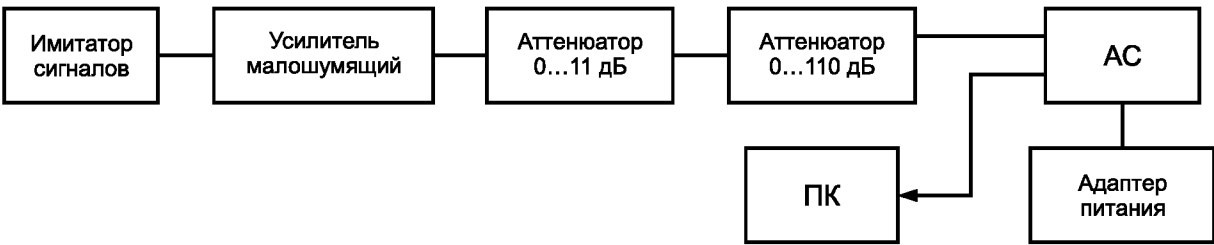
Рисунок Д.3 — Схема определения чувствительности модуля ГНСС
