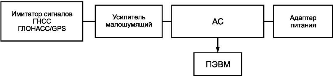
Рисунок Д.1 — Схема испытательного стенда
