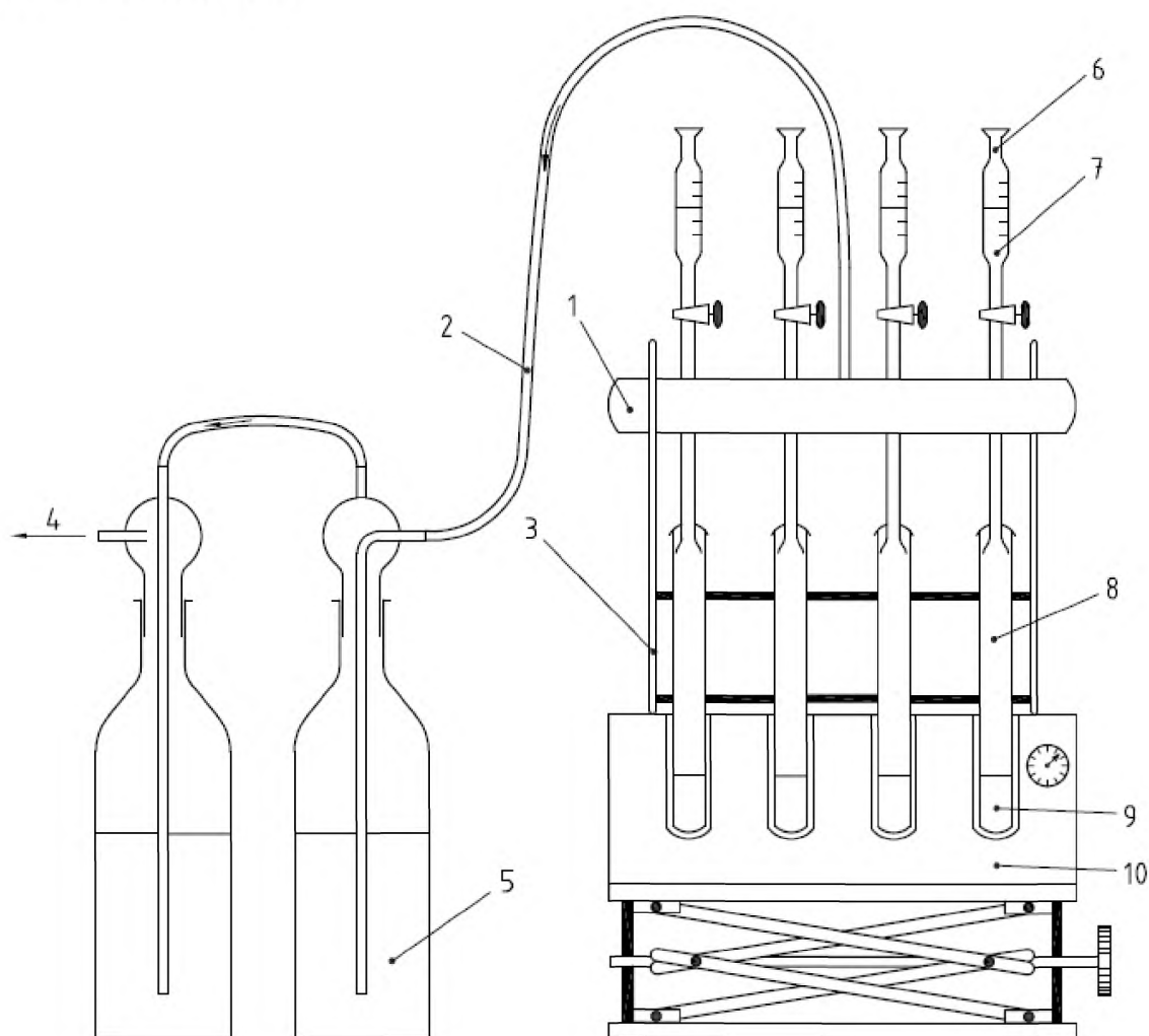
1 – вытяжной колпак; 2 – трубка для отсасывания кислотных паров; 3 – штатив; 4 – к отсасывающему насосу; 5 – раствор гидроокиси натрия; 6 – капельная воронка; 7 – перекись водорода; 8 – пробирка для разложения; 9 – образец для испытаний в концентрированной серной кислоте; 10 – нагревательный блок
