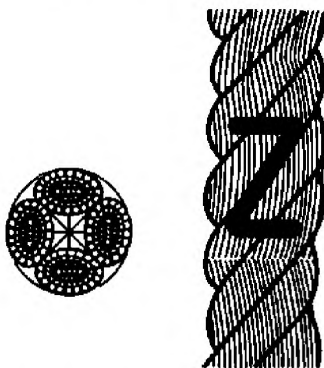
Рисунок 2 – Конфигурация 4-рядного (shroud-laid) каната (тип B)
