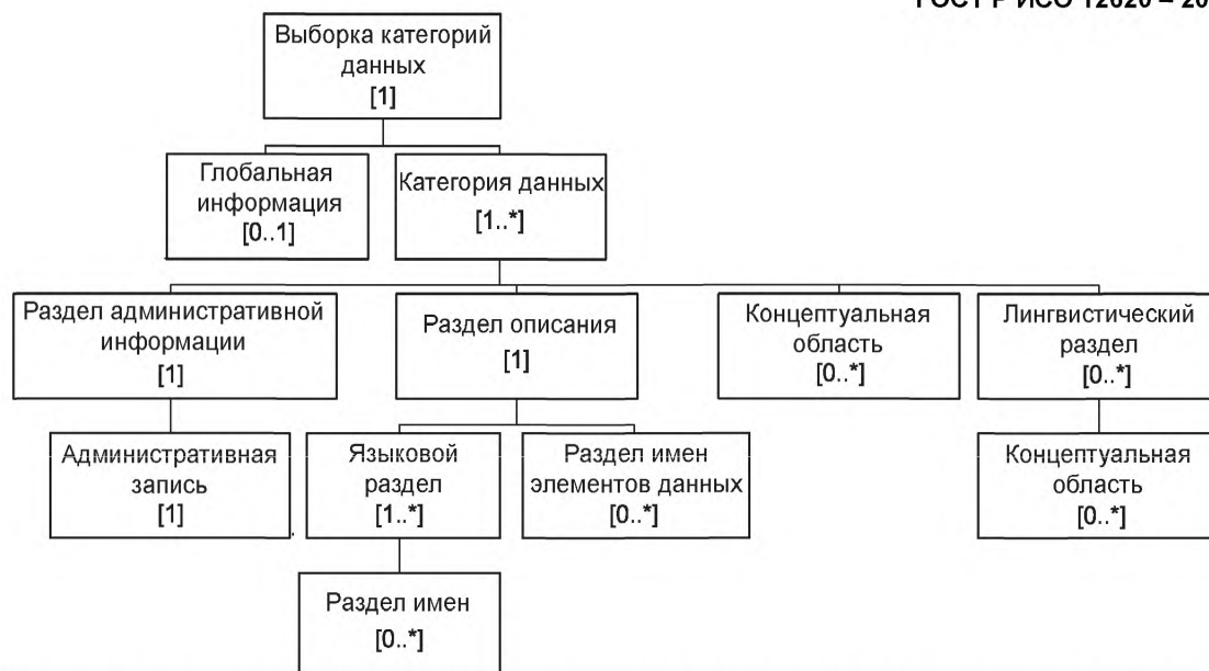
Рисунок 7 – Модель данных в основе DCIF
