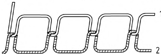
1 – игловая нитка, 2 – шпулечная нитка
