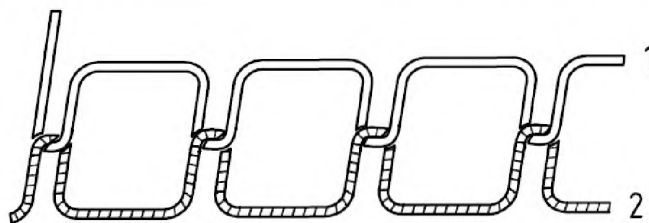
1 – игловая нитка; 2 – шпулечная нитка
