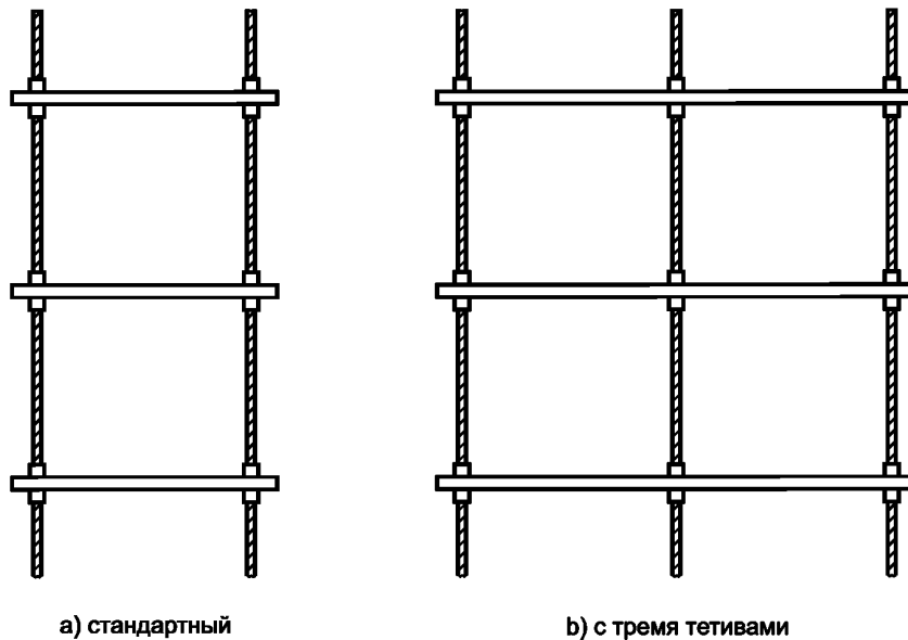
Рисунок 1 — Штурмтрапы
