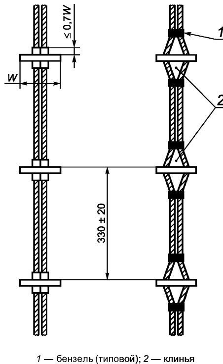
Рисунок 4 — Конструкции штурмтрапа с использованием механических зажимов (слева) и бензелей и клиньев (справа)
