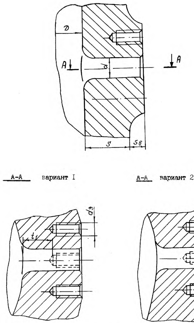
Рисунок 4.4 – Размещение резьбовых гнезд для крепежных элементов
