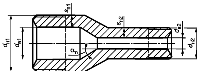
Рисунок 7 — Конический переход (тип А)
