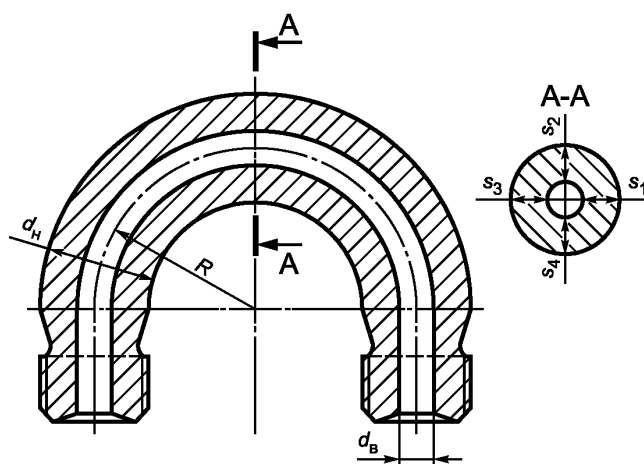
Рисунок 3 — Двойное колено трубопровода
