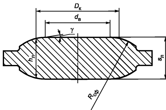
Рисунок 26 — Заглушка (тип В)
