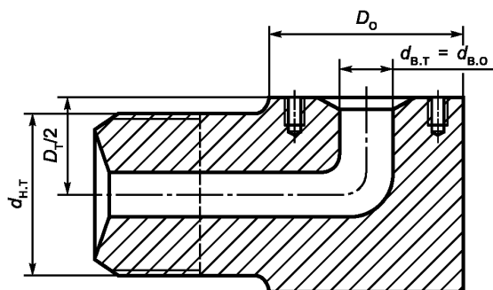
Рисунок 15 — Угольник (тип А)
