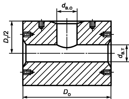
Рисунок 14 — Тройник (тип Д)
