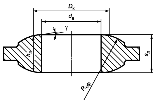
Рисунок 19 — Сферическая линза
