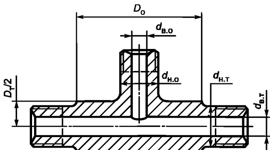
Рисунок 10 — Тройник (тип А)
