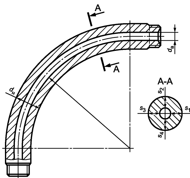
Рисунок 3 — Двойное колено трубопровода
