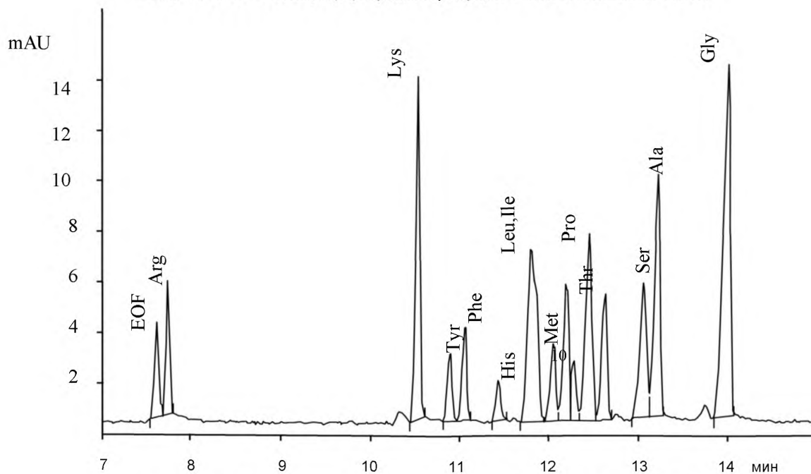
Рисунок А.1.2 – Электрофореграмма подготовленной пробы рыбной муки
