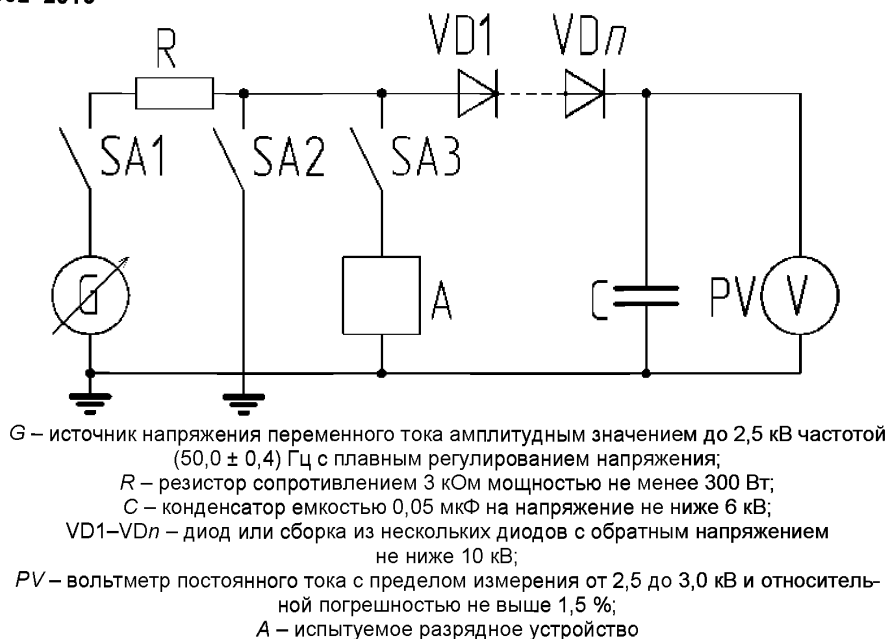
Рисунок 1 – Схема для проверки напряжения срабатывания разрядного устройства
