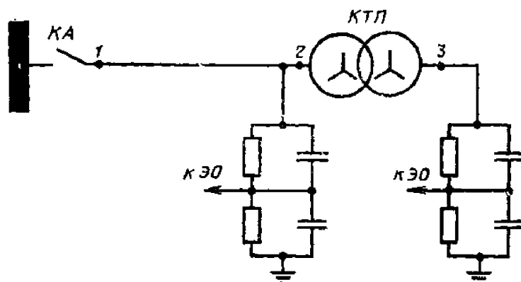
Схема коммутации низкого напряжения
