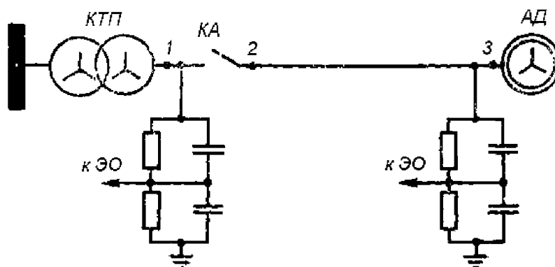
Схема коммутации низкого напряжения
