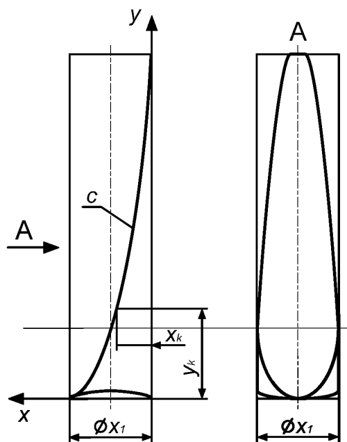
Рисунок 5— Стабилизатор
