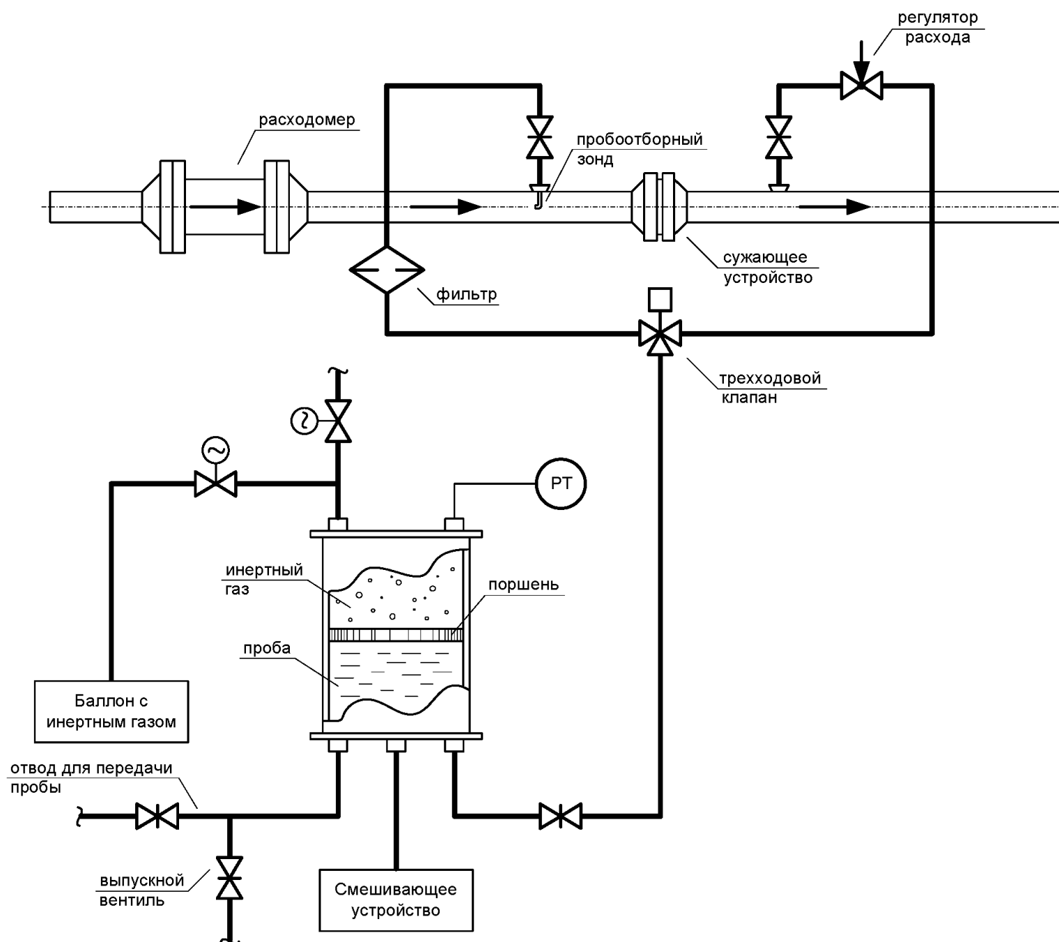
Рисунок 16 — Схема для автоматического отбора проб продуктов
