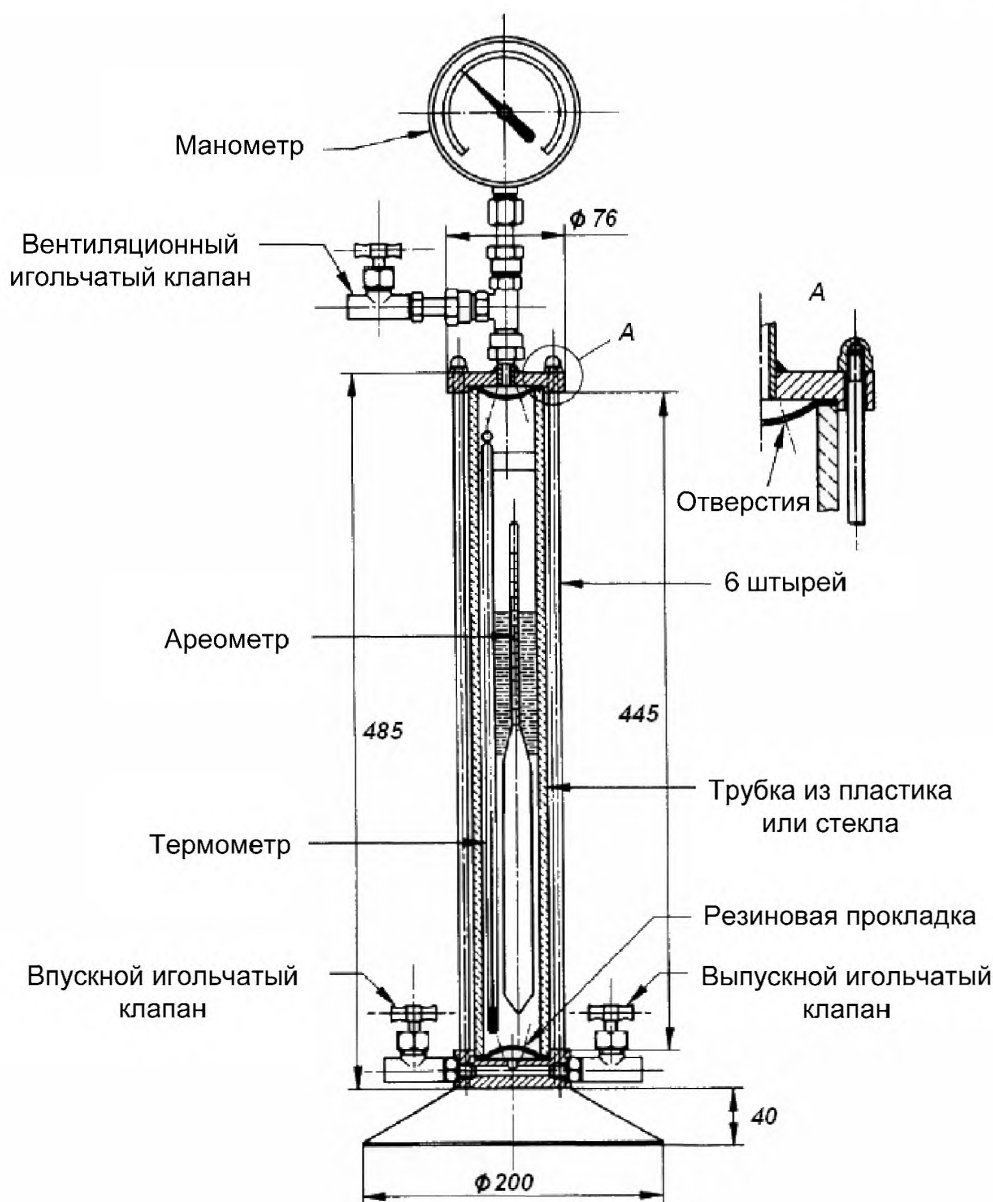
Рисунок 13 — Ареометр давления
