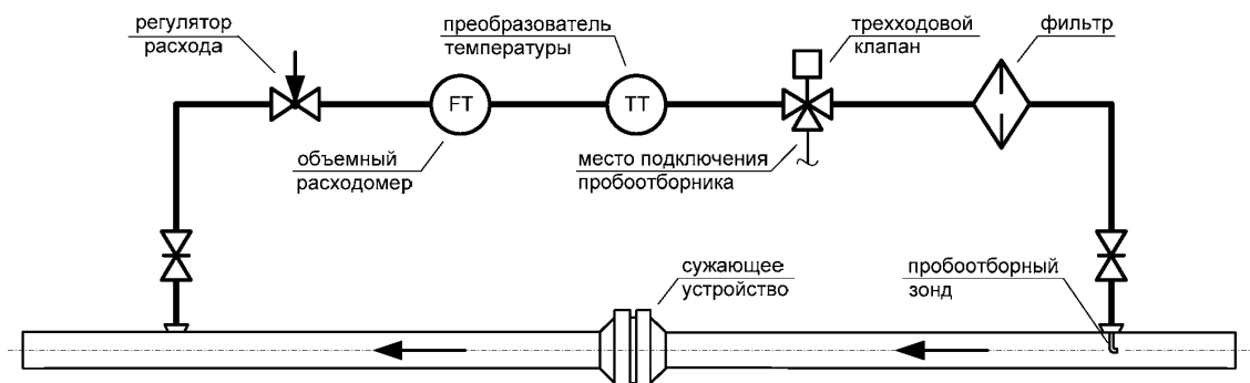
Рисунок 6 — Схема отбора проб с помощью сужающего устройства
