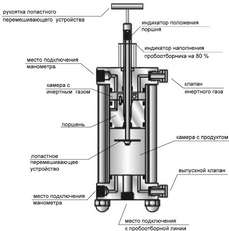
Рисунок 14 — Баллон постоянного давления поршневого типа
