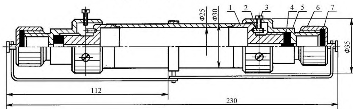
Рисунок 8 — Пробоотборник ПУ-400
