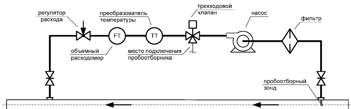
Рисунок 7 — Схема отбора проб с помощью насоса
