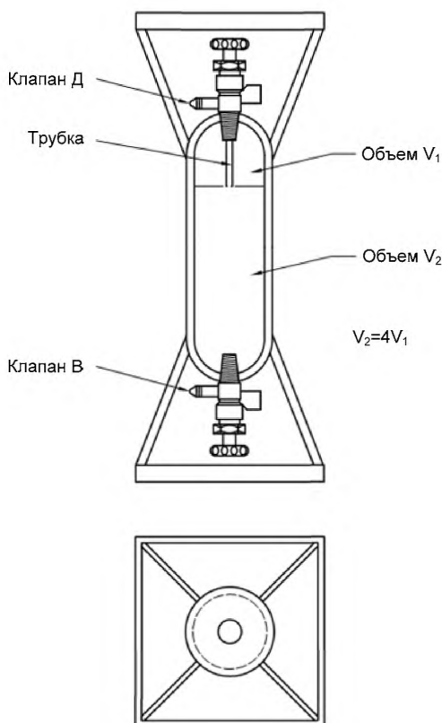
Рисунок 12. Пробоотборный контейнер с двумя клапанами
